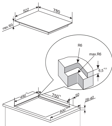
Montage ohne Lüftungsspalt vorne
