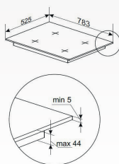
Montage ohne Lüftungsspalt vorne
