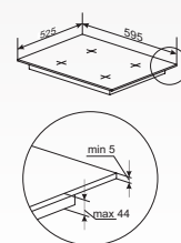
Montage ohne Lüftungsspalt vorne
